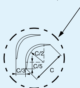
Detalle álabes de grosor aerodinámico
